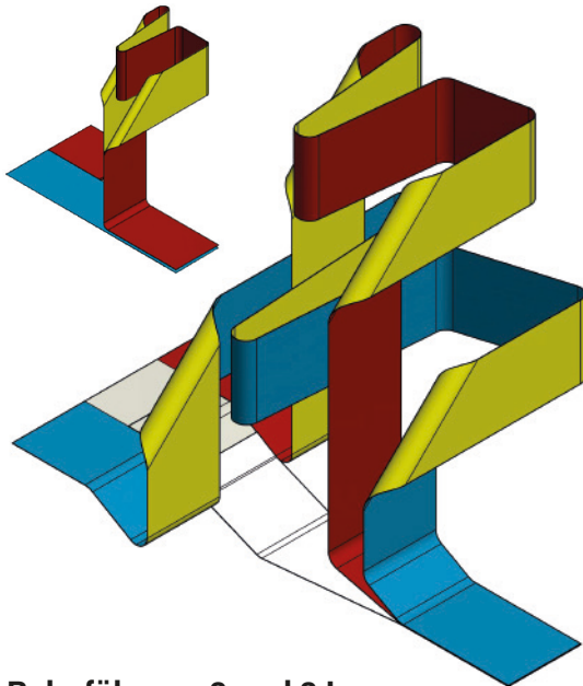
Bahnführung 2 und 3 Lagen
